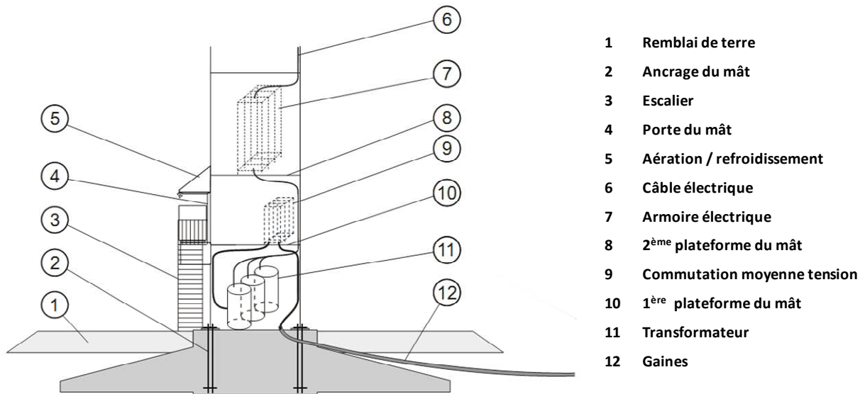
Figure 3 – Vue d'ensemble du pied de mât
