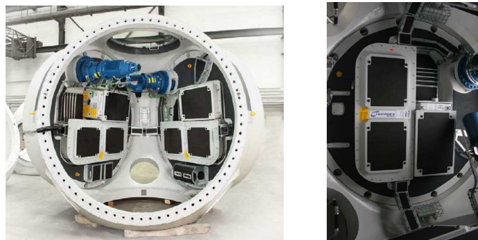
Figure 7 – Moyeu d'une éolienne Nordex Version Gamma : Détail
