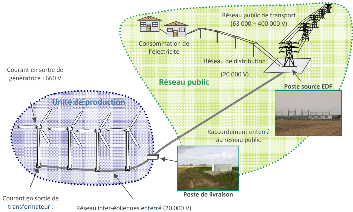
Figure 1 – Principe de fonctionnement d'un parc éolien
