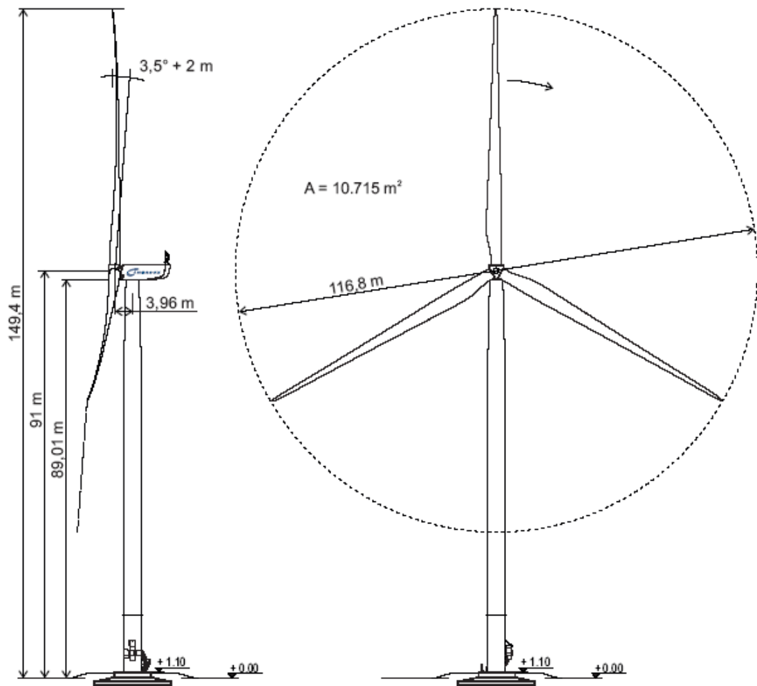
Figure 2 – Vue d'ensemble de l'éolienne Nordex N117/2400, hauteur de moyeu 91 (transformateur interne)
