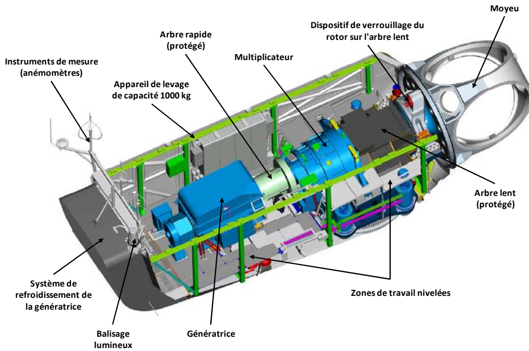
Figure 5 – Nacelle d'une éolienne Nordex Version Gamma
